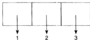
图 3-16 数组的概念
