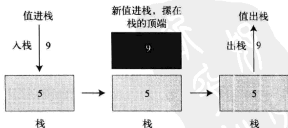
图 2-8 栈的构造
