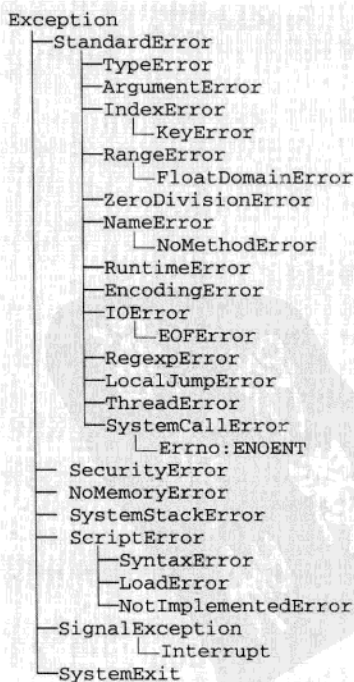
图 11-13 Ruby 的异常类层次结构图
