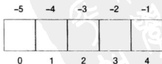
图 3-17 数组的下标
