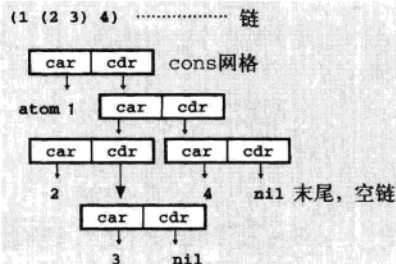
图 14-2 Lisp 的链
